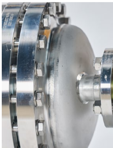
Výměník Green Hydrogen Systems, zdroj: Miloš Šálek
